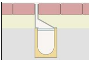
Afdekking asymmetrisch
