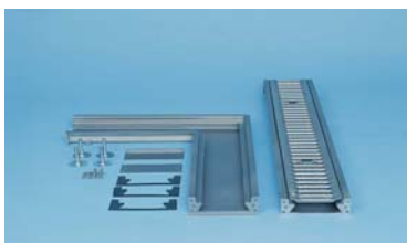
Gooitelement opbouw
